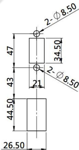
PANEL CUTOUT MS460-1-1
